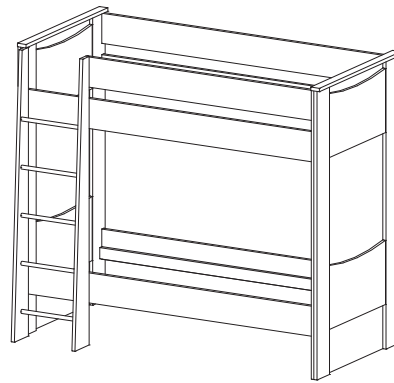
FERDA 11 L+P Patrová postel 900×2000 1133×1826×2095
