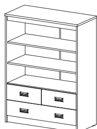
FERDA 61 Skříňka policová se zásuvkami 1000×1342×470
