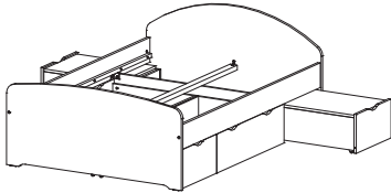
PEDRO K 73 Postel 1400x2000 se 6 úložnými prostory 1460x824x2046
